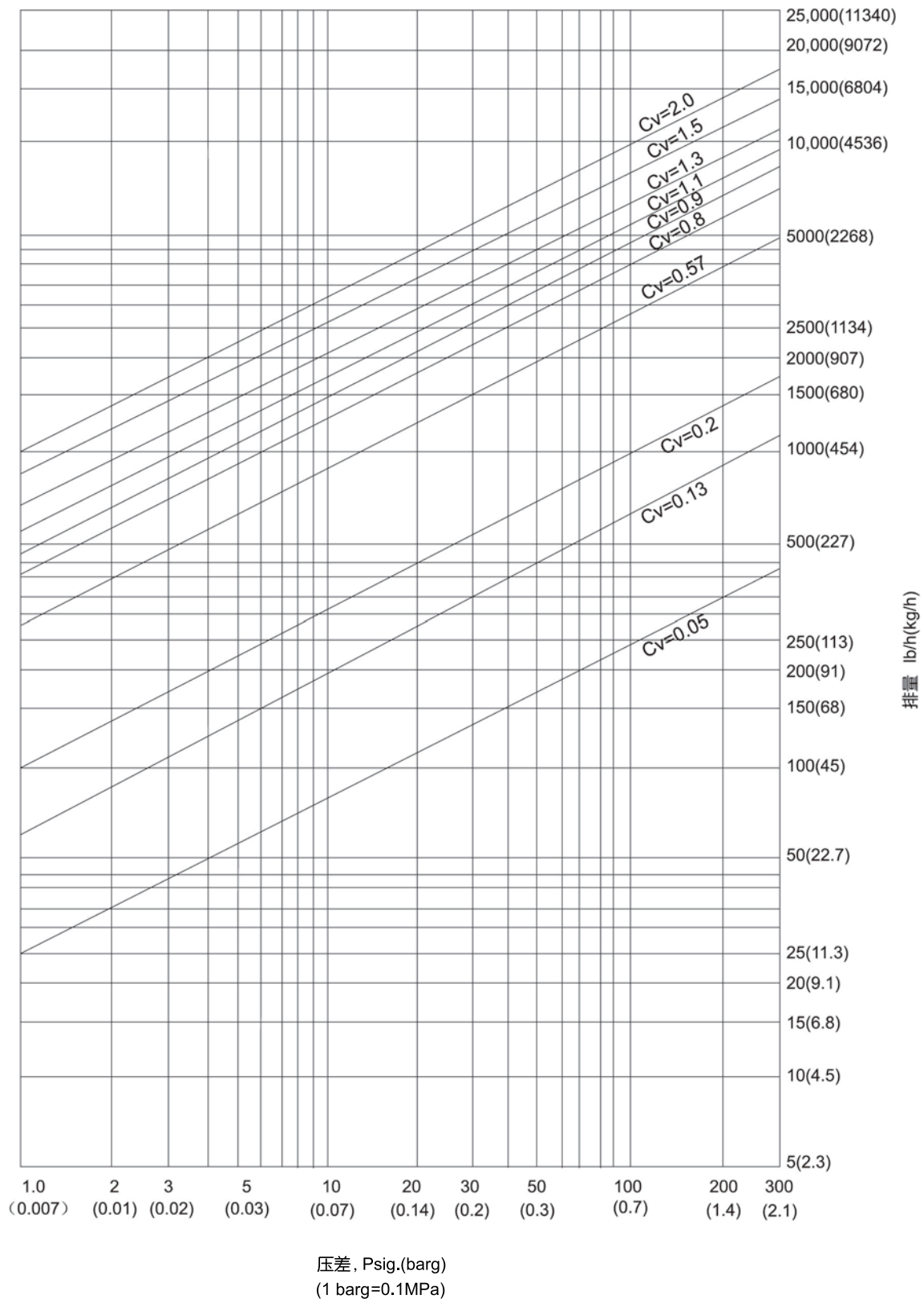
ASDV/CSDV 系列排量图
